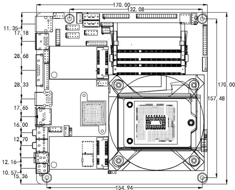
ITX-D81 VER:1.0 主板尺寸图
