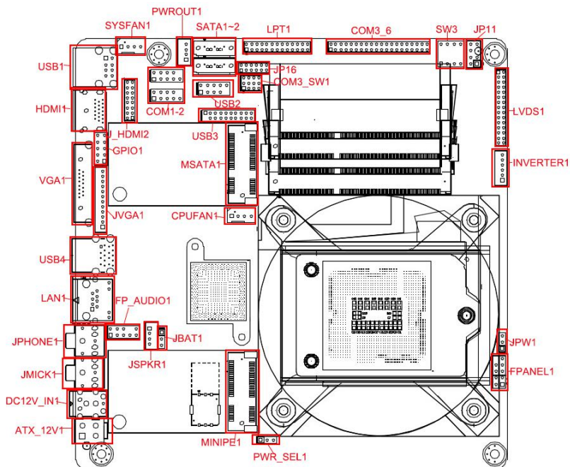
ITX-D81 VER:1.0 主板接口位置示意图
