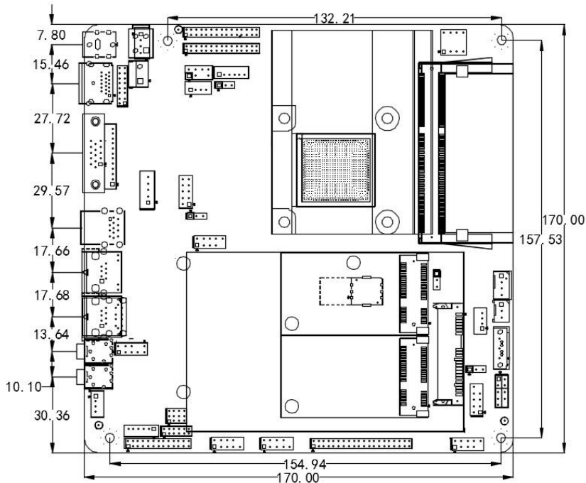
ITX-B190 VER1.1 尺寸图
