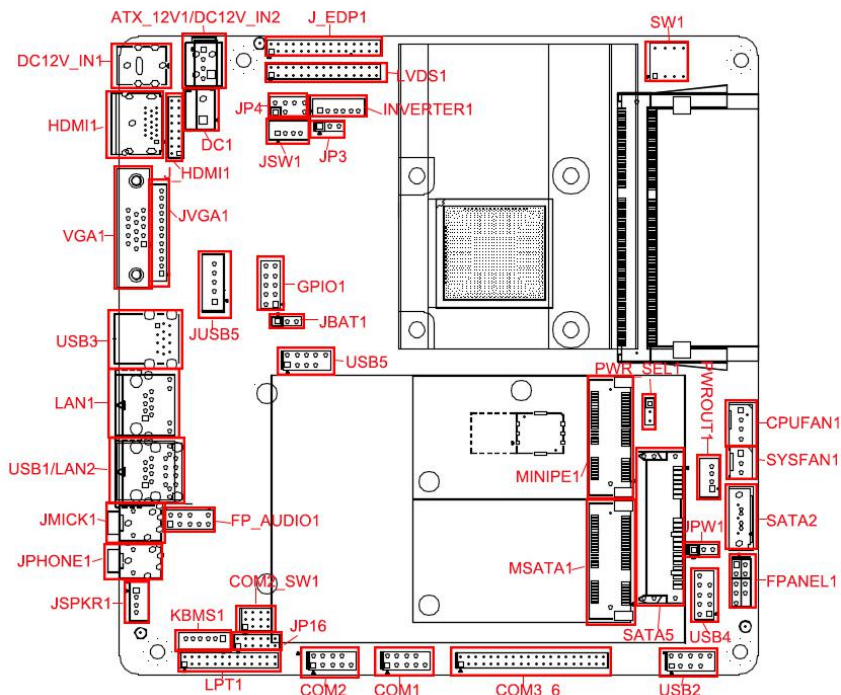
ITX-B190 VER:1.0 接口位置图
