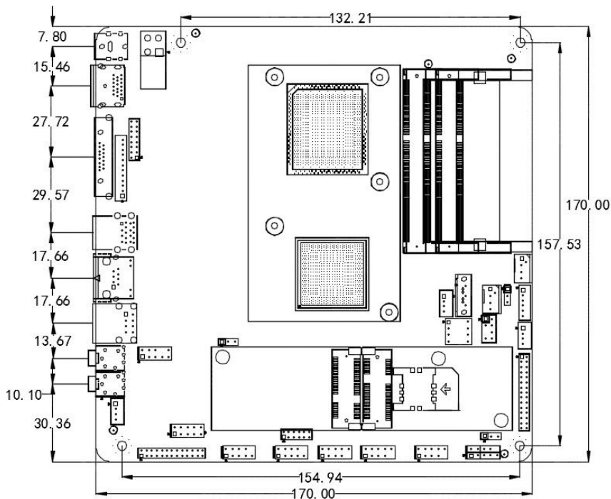
ITX-B530 VER:1.0主板尺寸图
