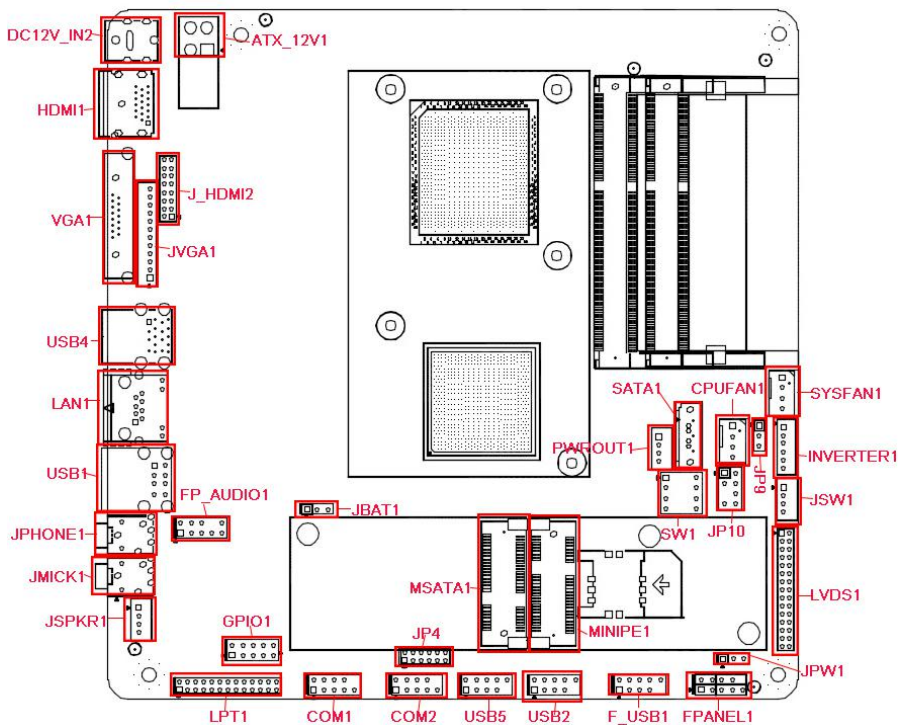
ITX-B530 VER:1.0主板接口位置示意图
