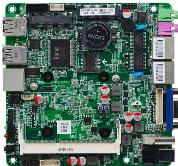
图一：STX-N39_19 VER:1.2A主板正面图
