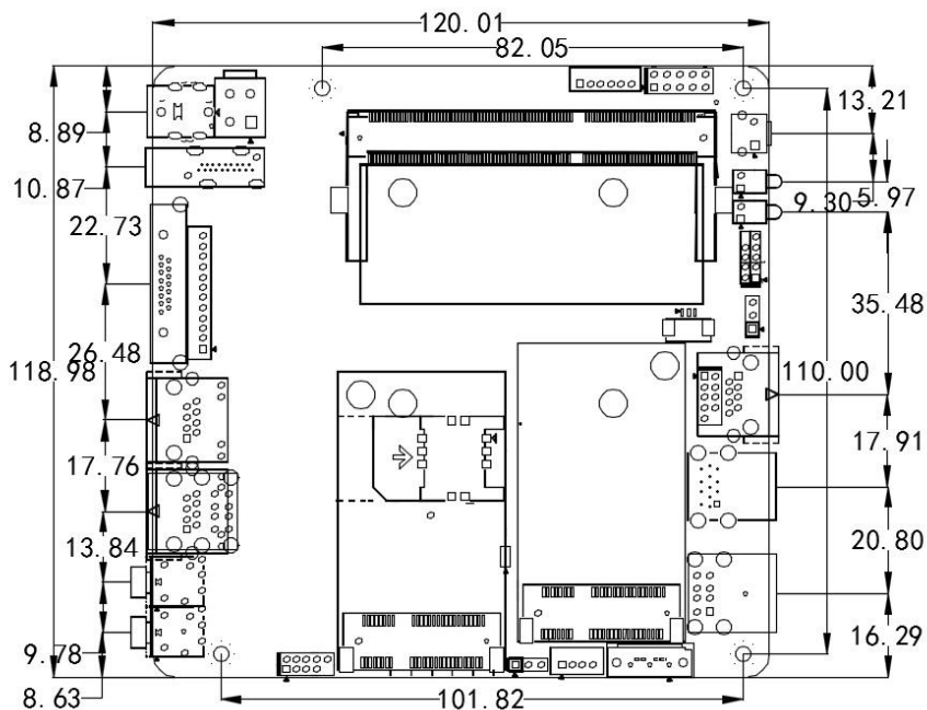
STX-N39 VER:1.2A 尺寸图
