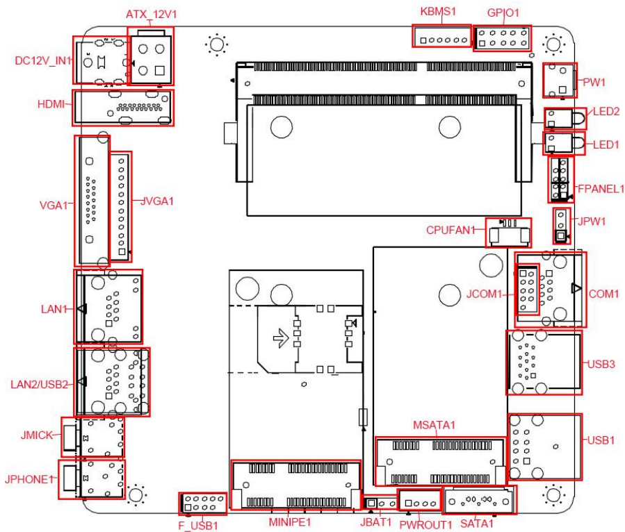
STX-N39 VER:1.2A接口位置示意图
