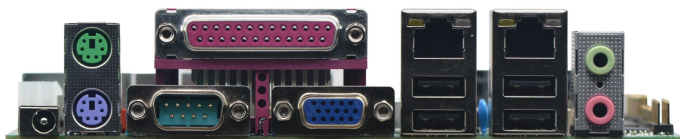
图二：ITX-M51_D926L VER:1.5A 主板 IO 图
