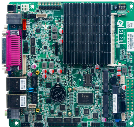
图一：ITX-M51_D926L VER:1.5A 主板正面图
