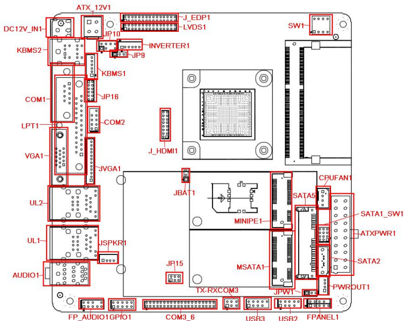
ITX-M51 VER:1.5A 接口位置图
