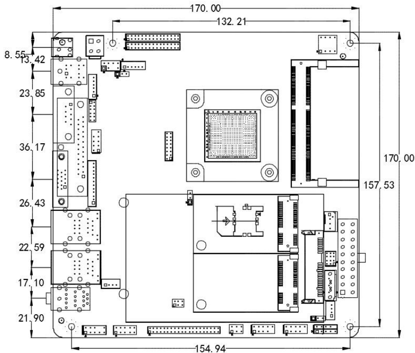
ITX-M51 VER:1.5A尺寸图
