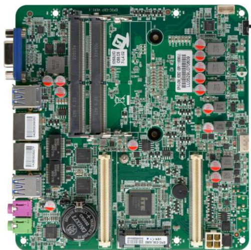
图一：EPIC-C58 VER:1.1 主板正面图
