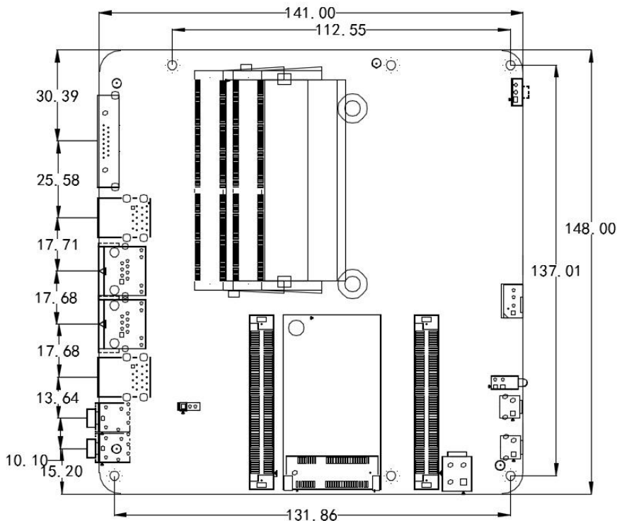
EPIC-C58 VER:1.1 尺寸图
