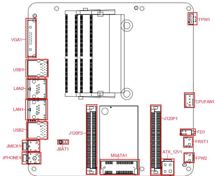
EPIC-C58 VER:1.0 接口位置图
