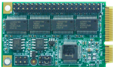
图三：TPM-4COM扩展板正面图
