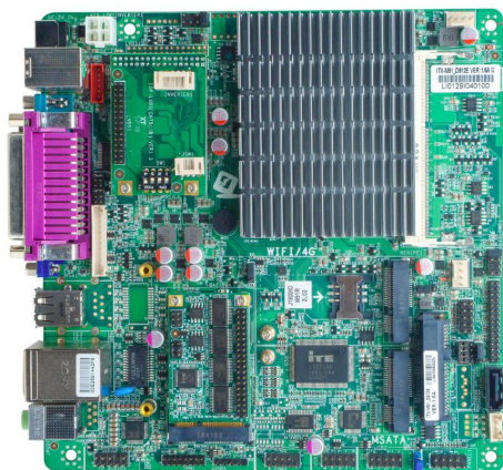
图一：ITX-M51 VER:1.6A搭配小板正面图
