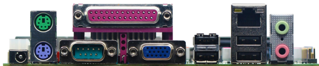
图二：ITX-M51_D912L VER:1.6A 主板 I/O 图
