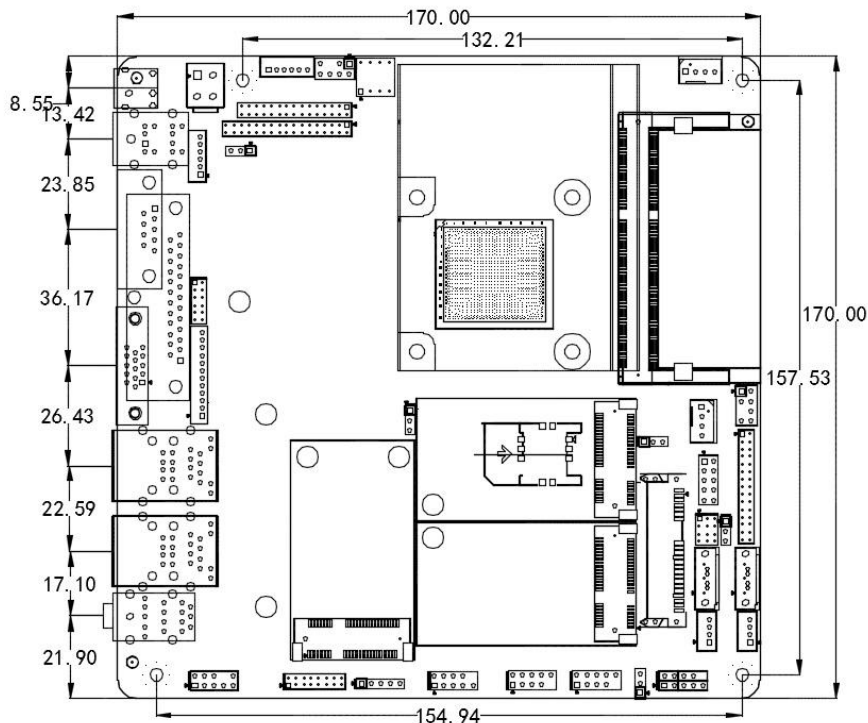
ITX-M51 VER:1.6A 尺寸图
