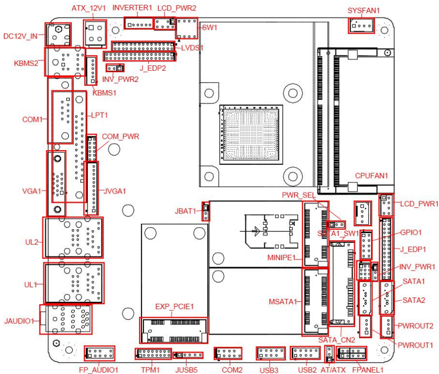
ITX-M51 VER:1.6A 接口位置图
