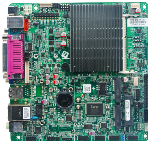
图一：ITX-M51_D912L VER:1.6A 主板正面图
