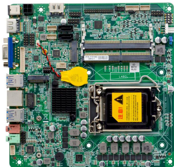
图一：ITX-Y310C VER1.0 正面图
