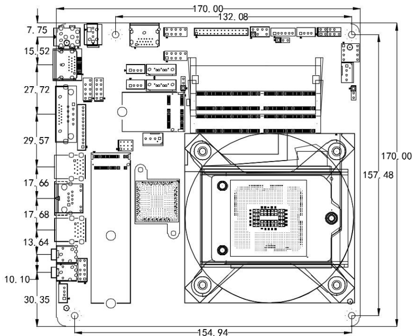
ITX-Y310C VER1.0 尺寸图
