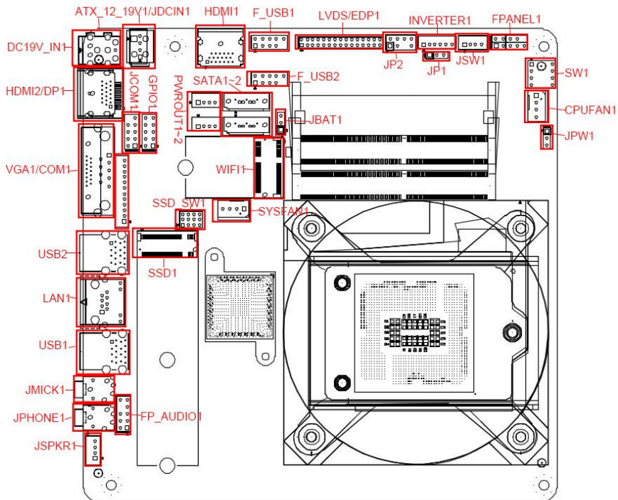
ITX-Y310C VER1.0 接口位置图
