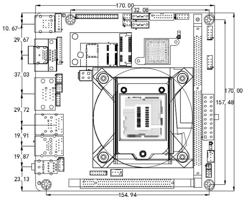
ITX-H81R1 VER:1.0 尺寸图
