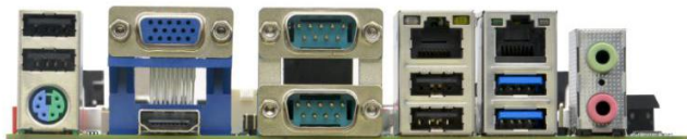
图二：ITX-H81R1 VER:1.0 主板 I/O 接口图
