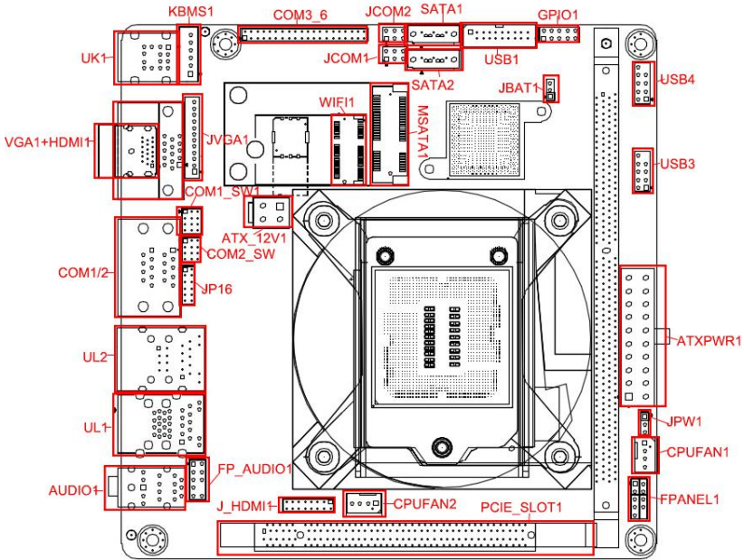
ITX-H81R1 VER:1.0 接口位置图
