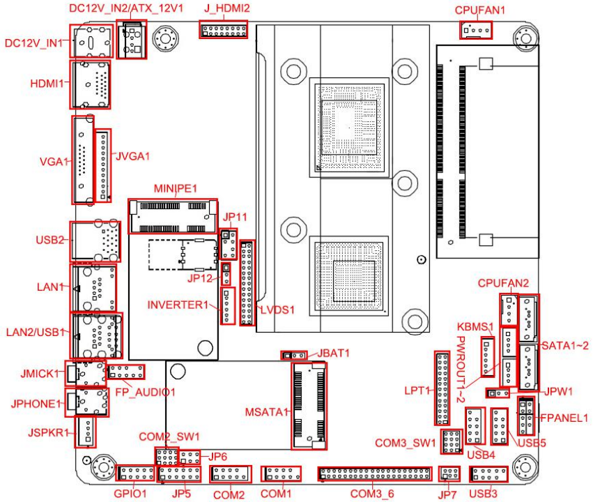
ITX-B330 接口位置图
