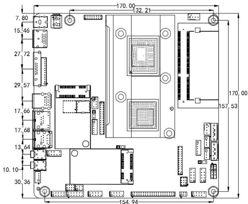
ITX-B330 VER:1.0 主板尺寸图
