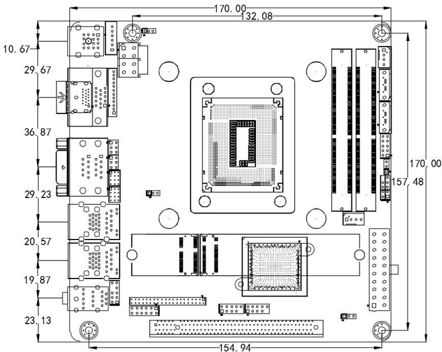
ITX-H610M1 VER:1.0 尺寸图
