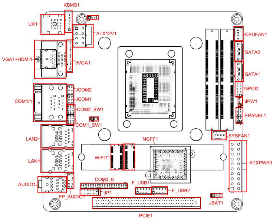
ITX-H610M1 VER:1.0 接口位置图
