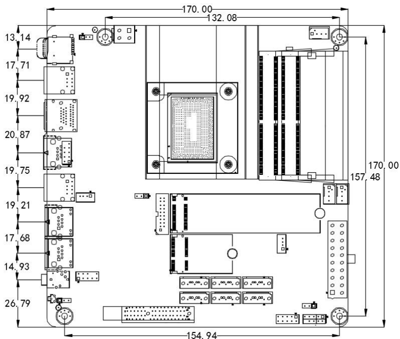
N510S6 VER:1.0 尺寸图
