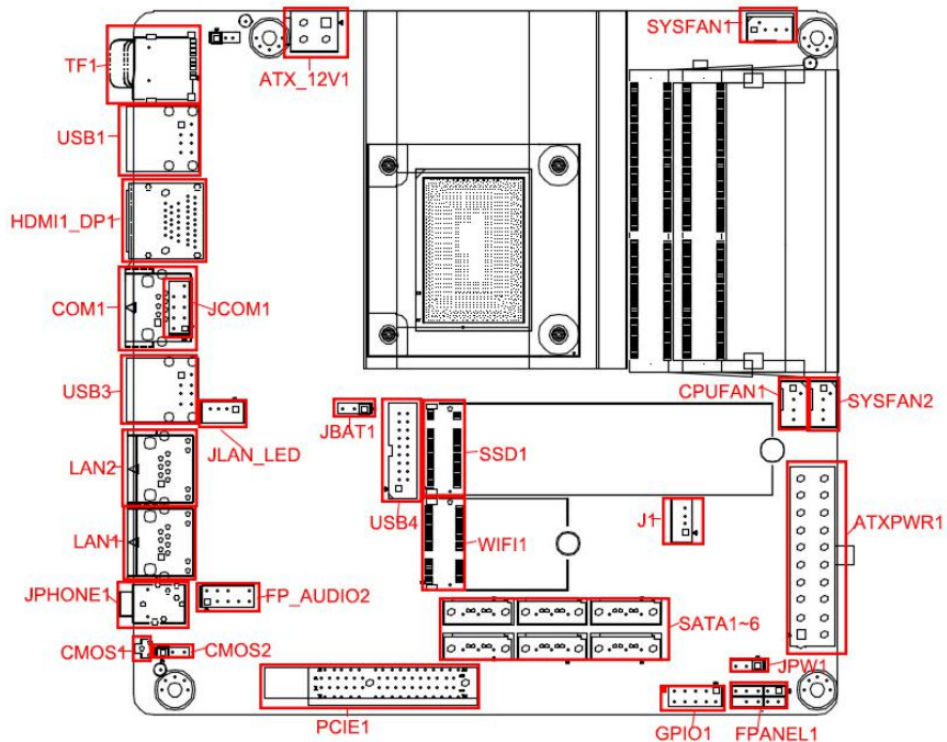
N510S6 VER:1.0 接口位置图
